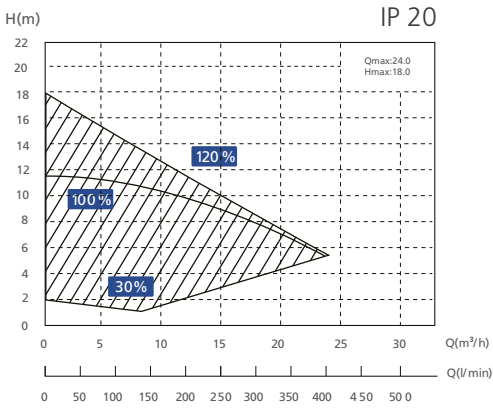
Leistungskurven:
