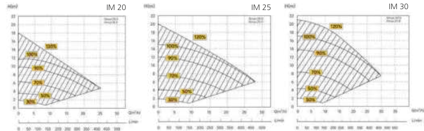
Leistungskurven:
